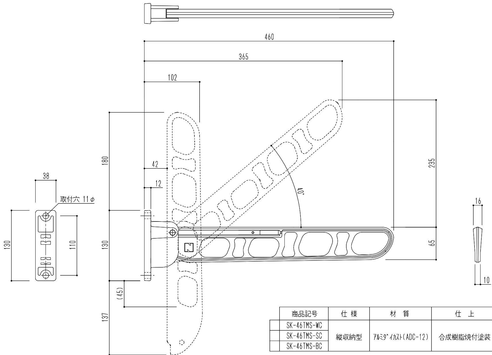
図面名 SK-46TMS-WC/-SC/-BC アルミ-物干金物(縦収納型)
